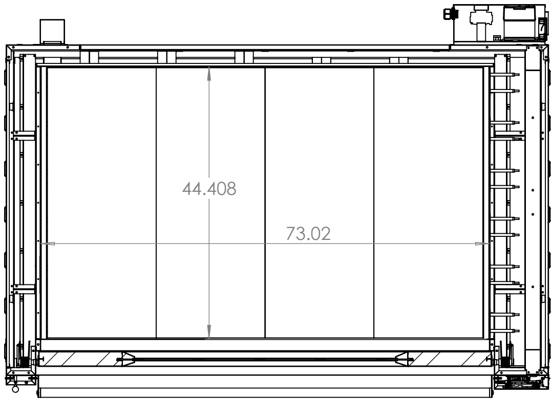
SECTION A-A SCALE 1 : 16
